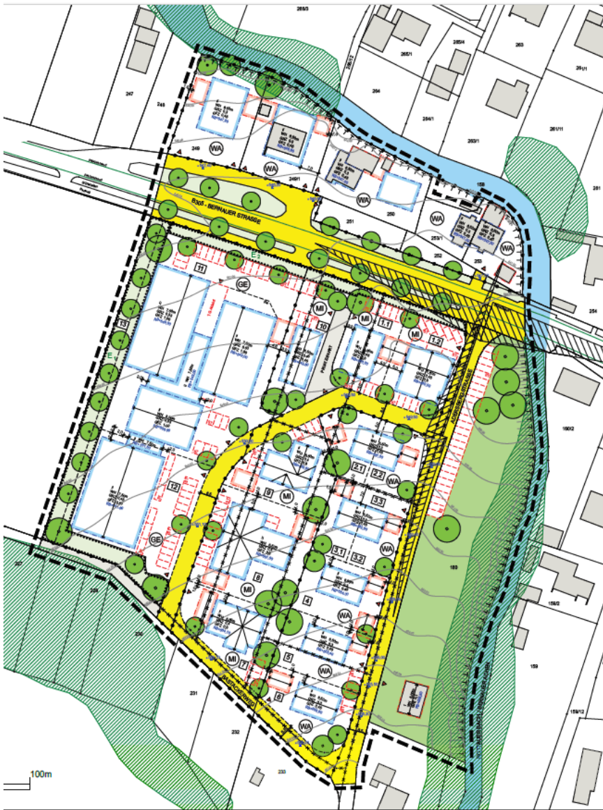
Plan Bauungsplan:
